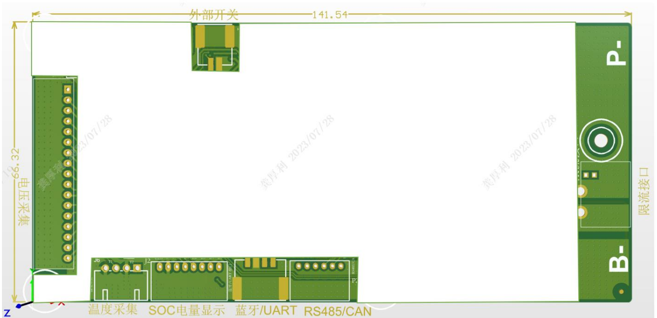
(图 3 PCB 板布局与尺寸图)
