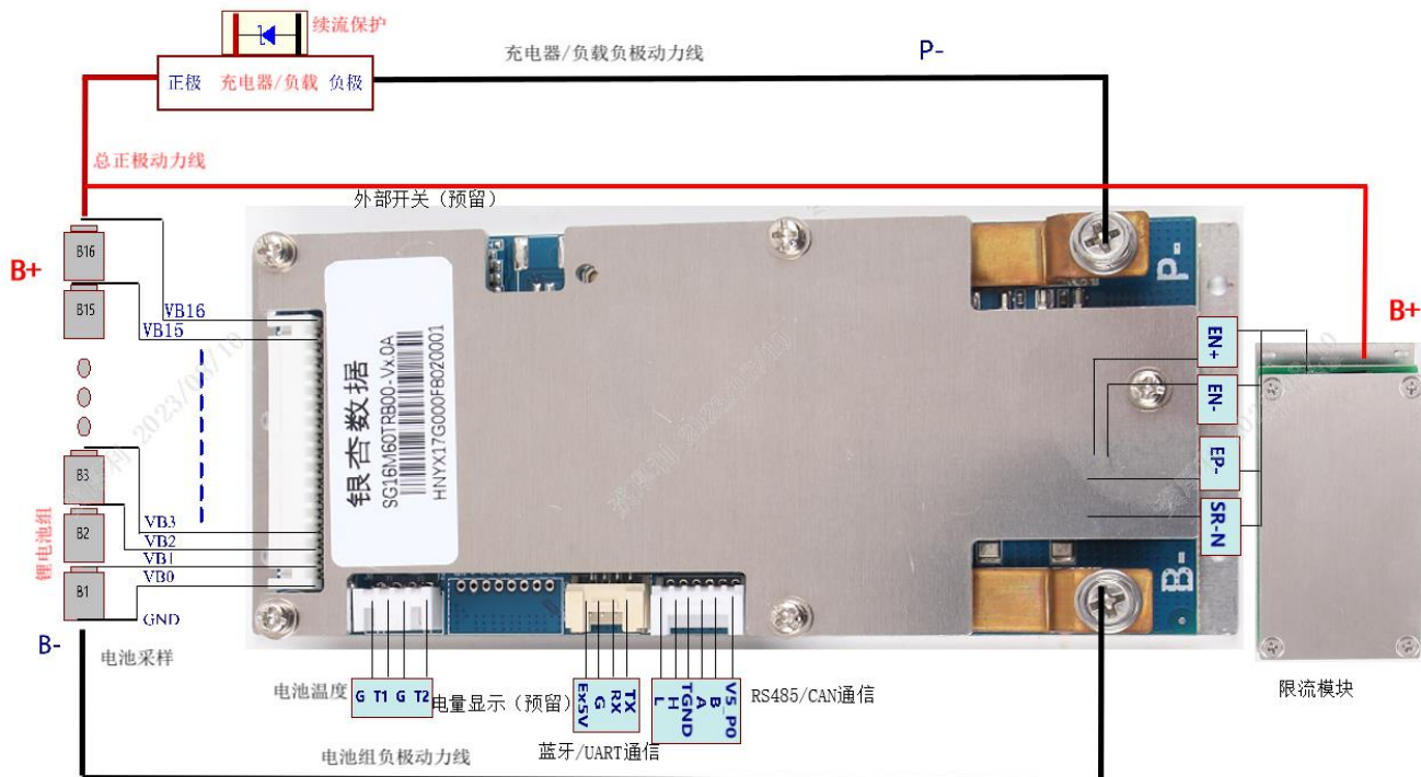
(图 2 充放电测试接线图)
