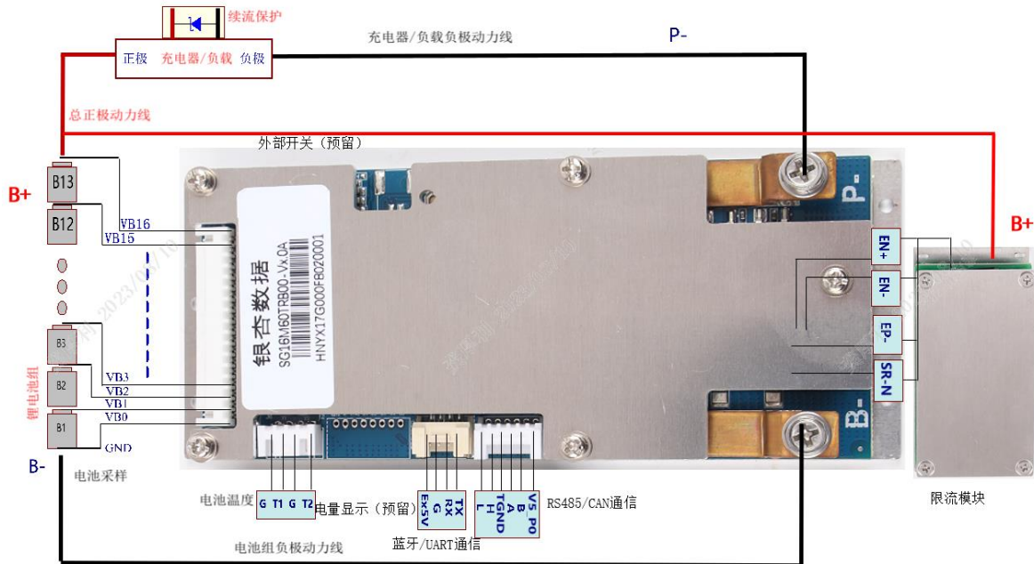
(图 2 充放电测试接线图)
