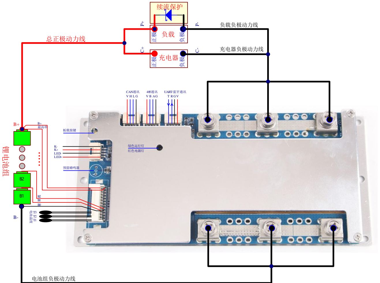
(图 2 充放电测试接线图)
